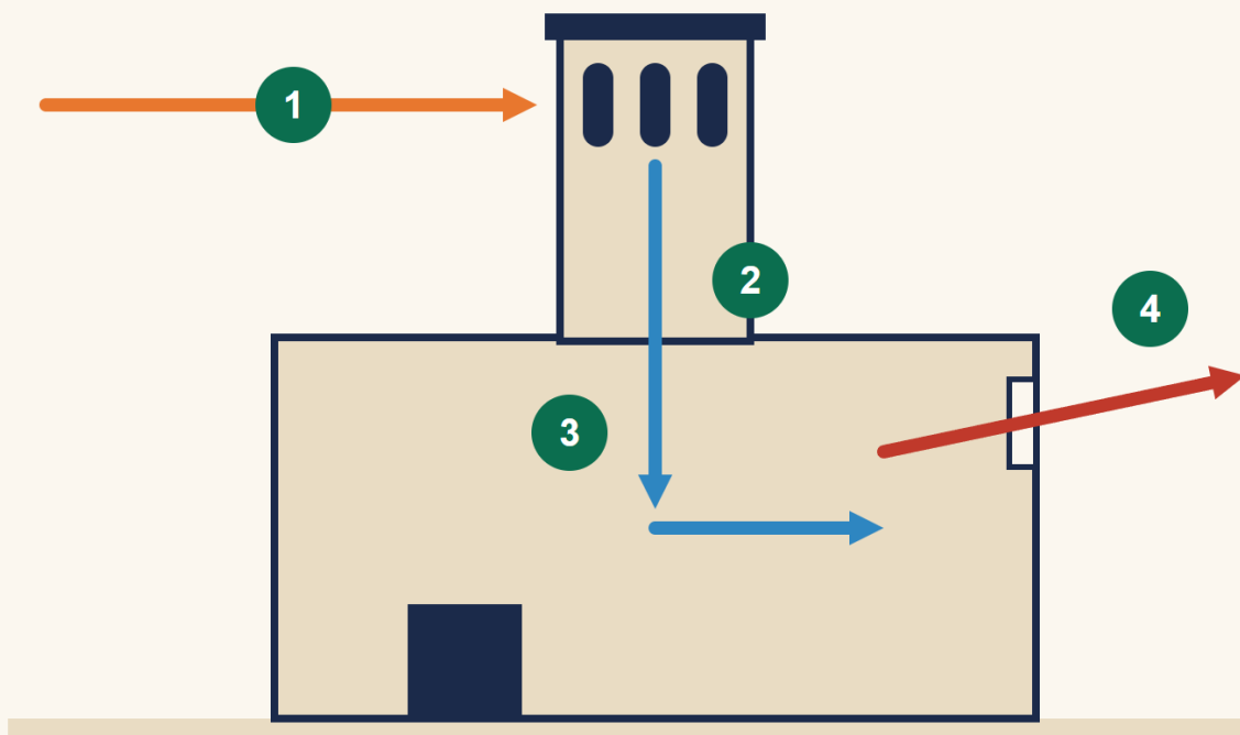
Tour à vent traditionnelle (coupe simplifiée)
